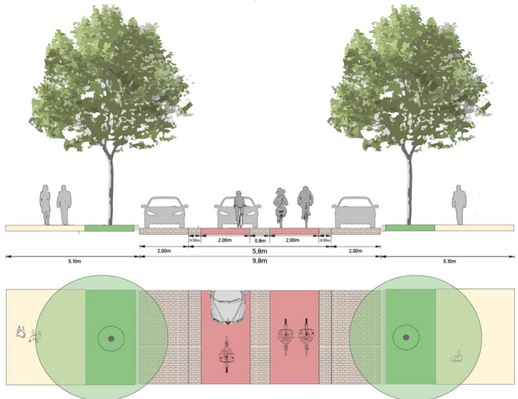
ABBILDUNG_14 | Entwurf für die Umgestaltung der Menzelstraße in eine Fahrradstraße
